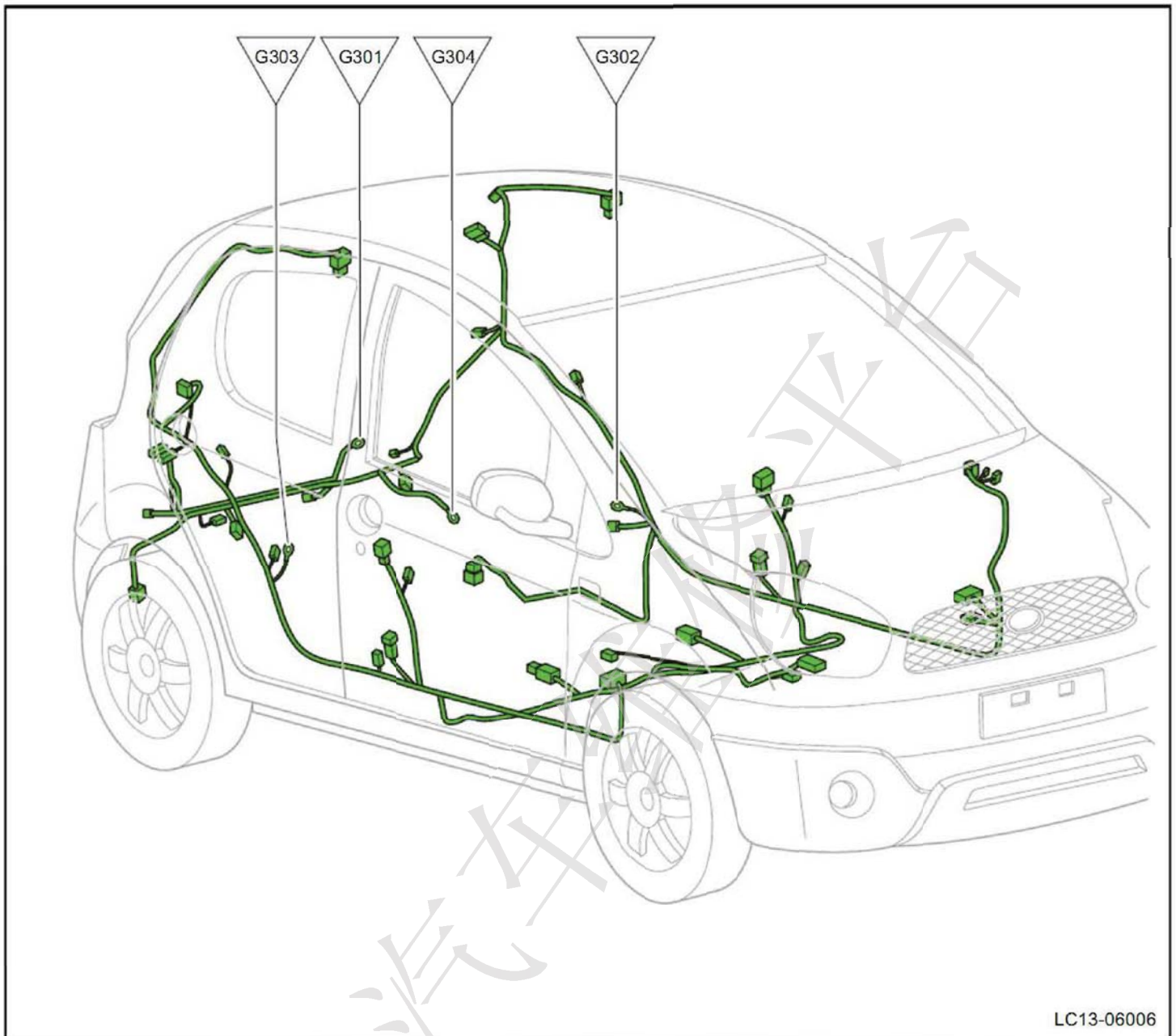
底板接地点布置图
