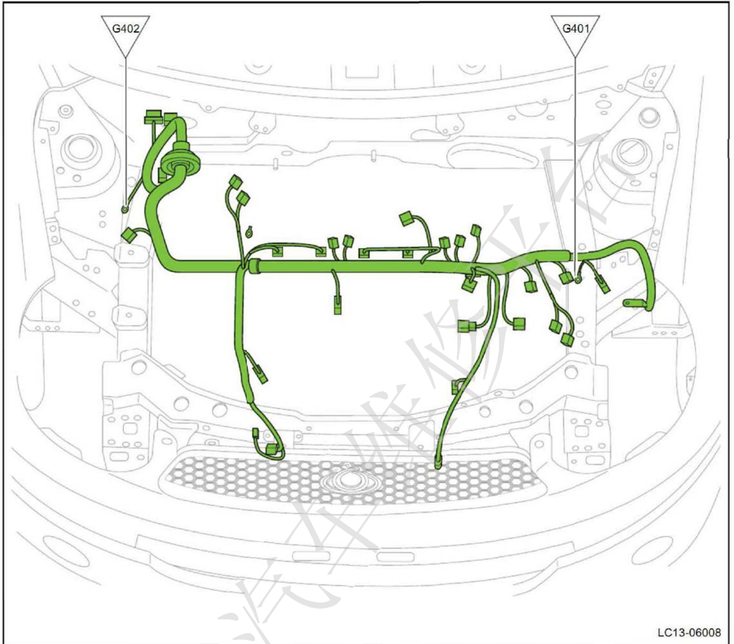
发动机接地点布置图
