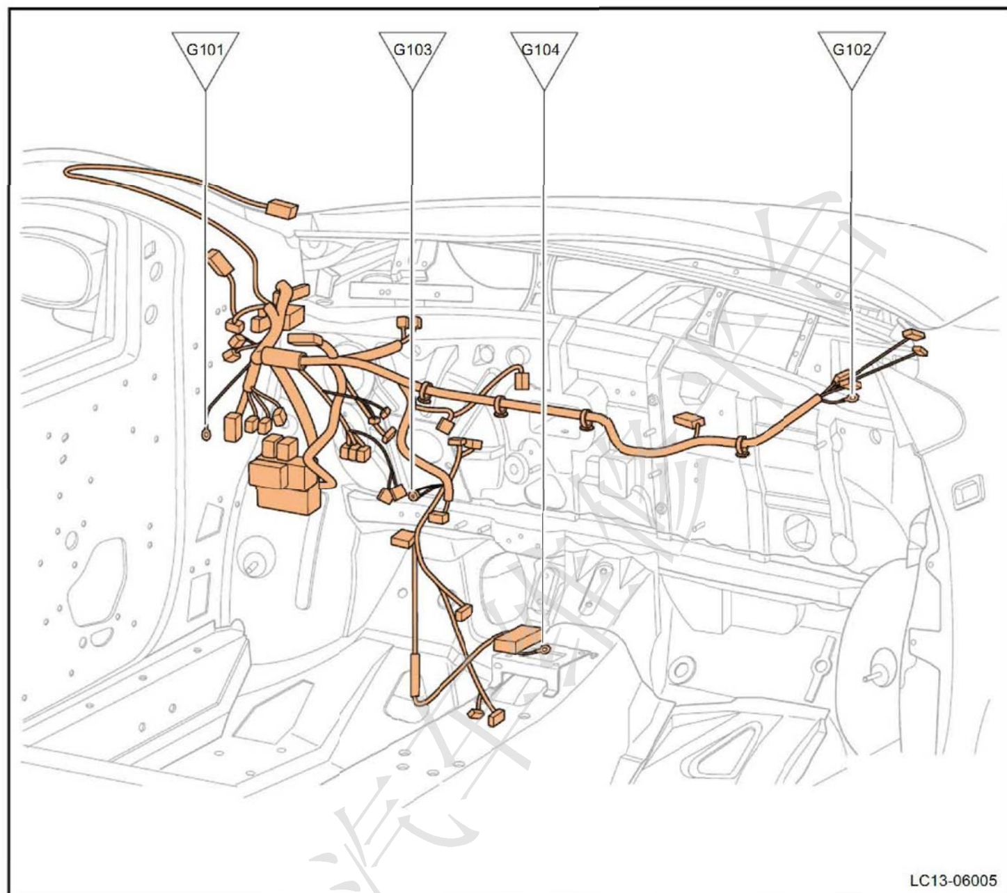
仪表接地点布置图
