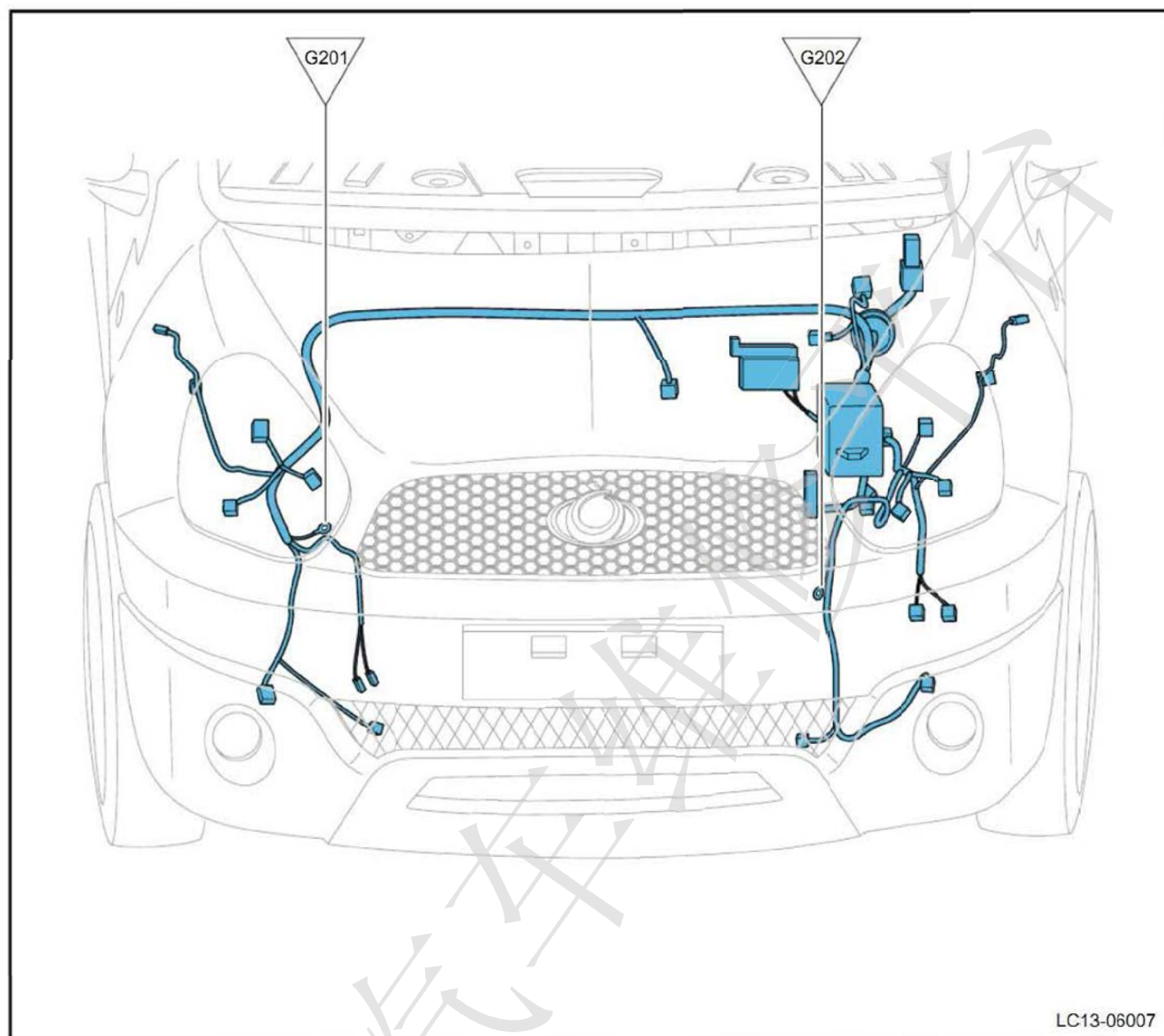
发动机舱接地点布置图
